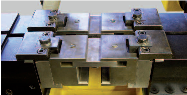
Spannbacken für nach oben offene C-Profile
