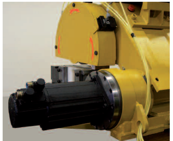
Vorschubeinheit mit Drehstrom Servomotor Bosch-Rexroth
