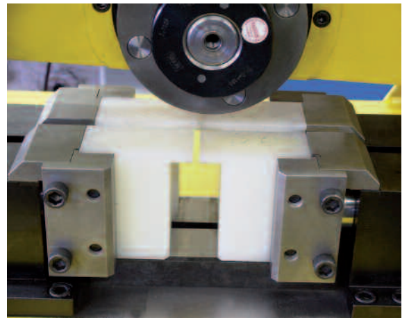
Doppelspannvorrichtung mit 4 hydraulischen Spannzylindern
