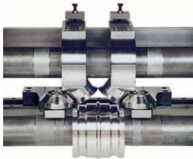
Seitenrollentisch in Winkelausführung
